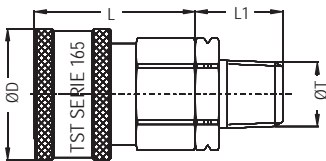
NPT (Taper) Male Threaded Shut-Off Socket Kupplungen mit Ventil und NPT Außengewinde
